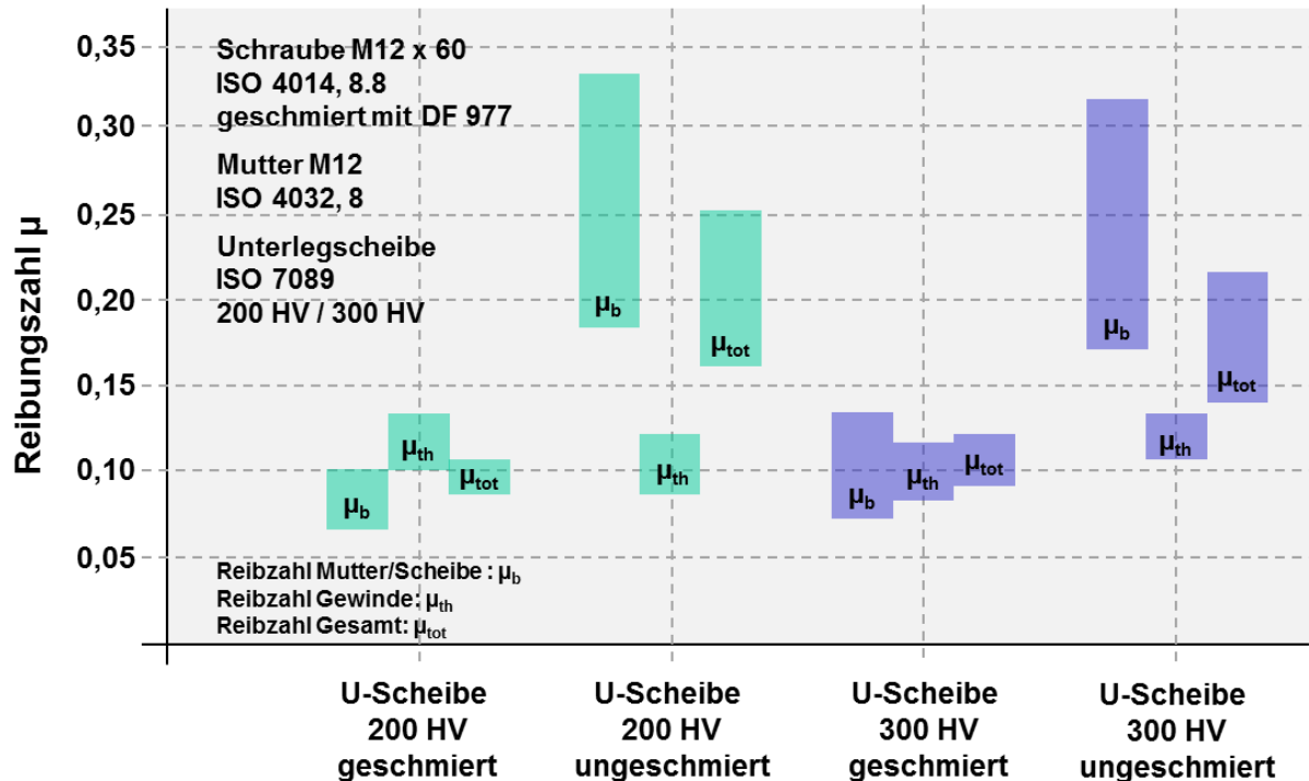
Abb.2: Vergleich der Reibzahlen des Gewindes, der Muttern-/ U-Scheibenauflage und des Gesamtreibwertes © Peter Thomsen, D-28211 Bremen
