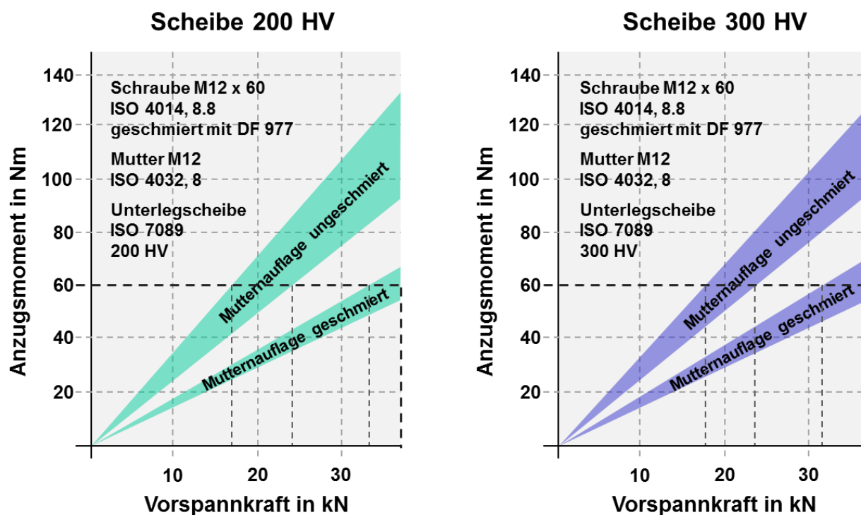
Abb.1: Schematische Darstellung der Ergebnisse der Drehmoment-/Vorspannkraftversuche © Peter Thomsen, D-28211 Bremen
