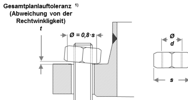
Abb.1: Gesamtplanauftoleranz t nach DIN EN ISO 4759-1
