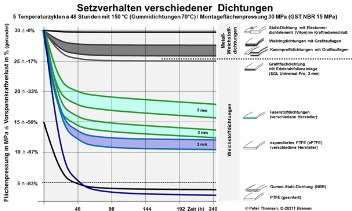
Abb.6: Setzverhalten verschiedener Dichtungen nach Lastzyklen unter Temperatur © Peter Thomsen, D-28211 Bremen
