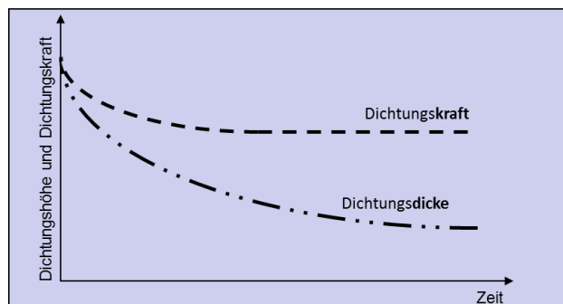
Abb.3: Schematische Darstellung der Kriech-Relaxation © Peter Thomsen, D-28211 Bremen
