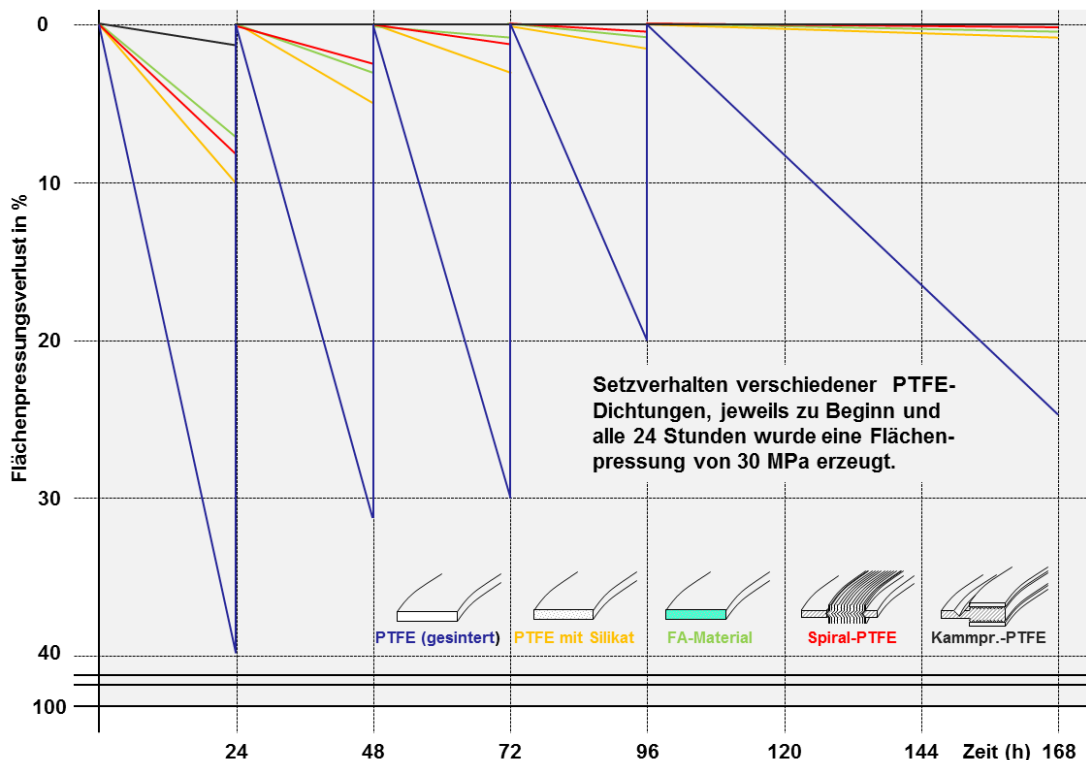
Abb.5: Setzverhalten verschiedener Dichtelemente © Peter Thomsen, D-28211 Bremen
