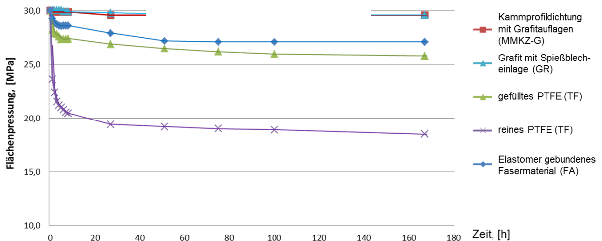
Abb.4 Darstellung der Messergebnisse © Peter Thomsen, D-28211 Bremen
