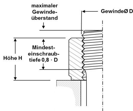
Abb.1: Darstellung der optimalen Mindesteinschraubtiefe bei Dehnschrauben
